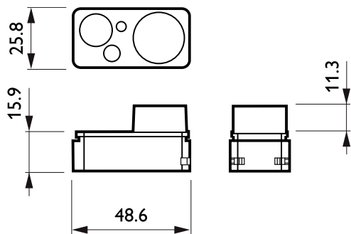
LRI1667/00 ActiLume G2 Indus Sensor H513
